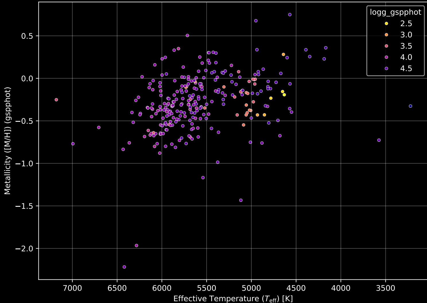
GALAH DR4 Field: [6917] Stellar Population Parameters (n= 274)
