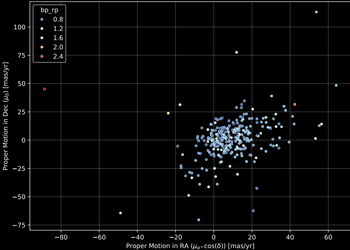
GALAH DR4 Field: [6917] Proper Motion Diagram (n= 274)
