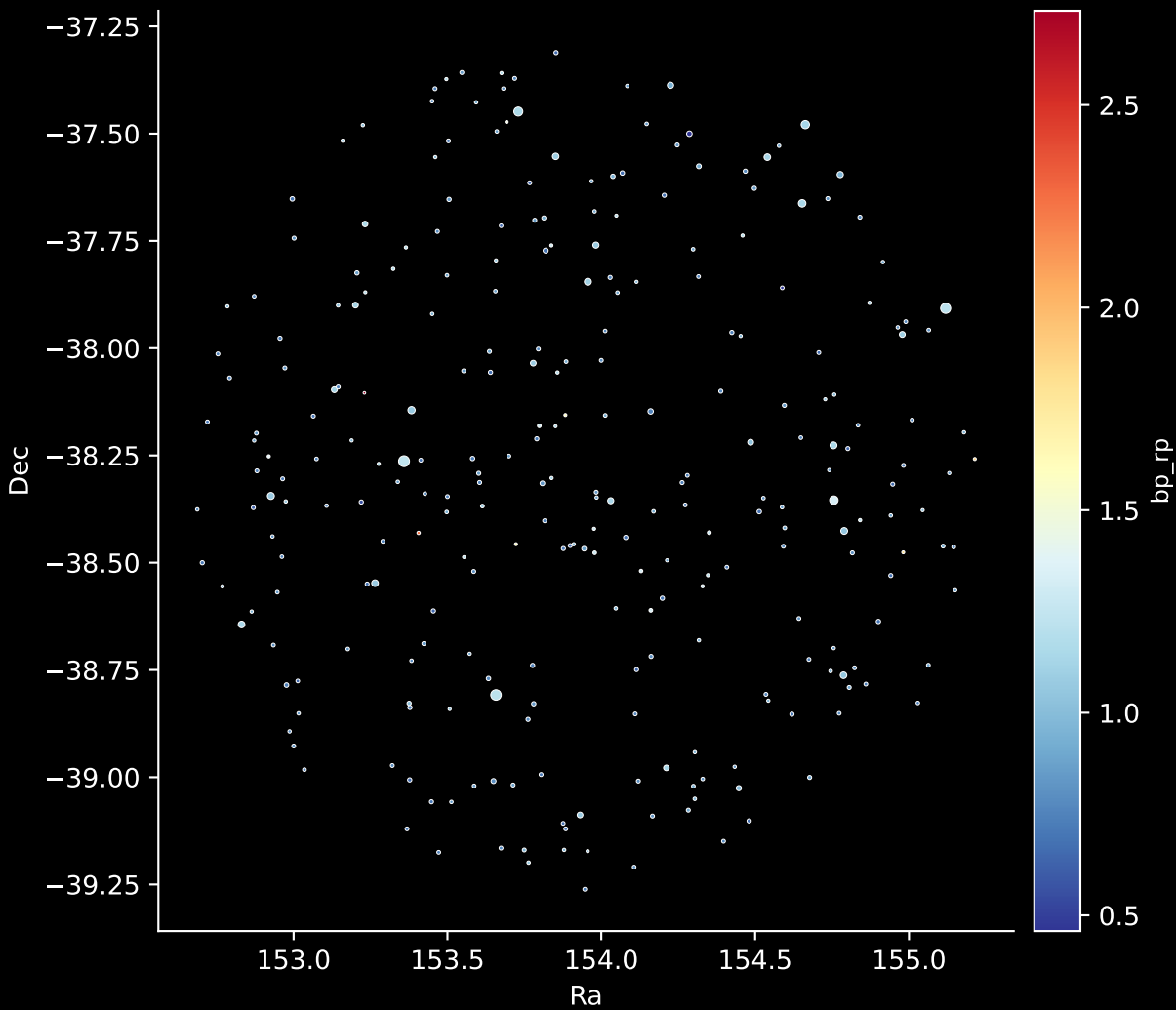
GALAH DR4 Field: [6917] Stars: 274
