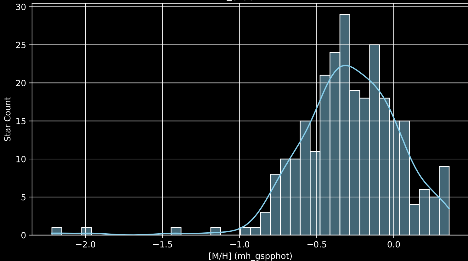
GALAH DR4 Field: [6917] [M/H] (mh_gspphot) (n= 271)
