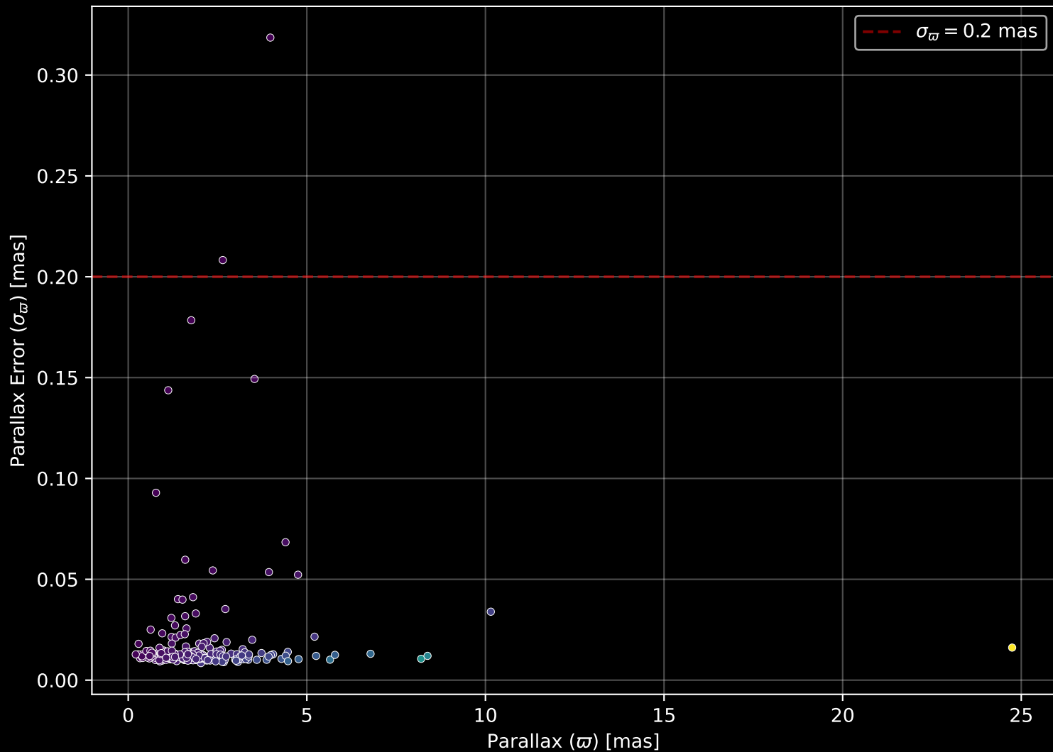
GALAH DR4 Field: [6917] Parallax Quality (n= 274)
